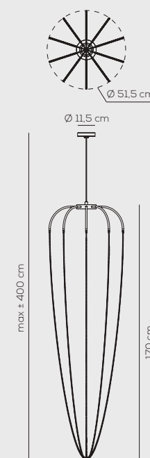
SP ALY 51 G kg 4,5 m² 0,11
