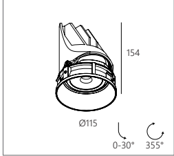
ROUND ØKIT
