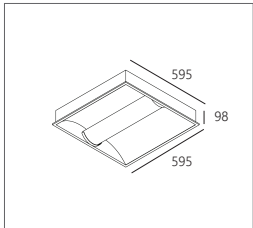
Diffuser 578 x 578
