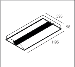
Metal Mesh 1178 x 578
